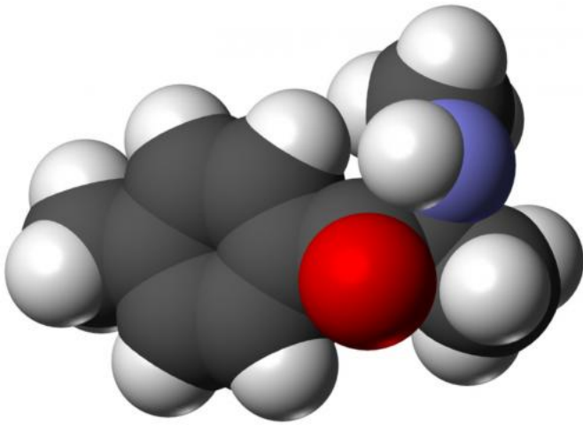
Mephedrone. Credit: Wikimedia Commons
